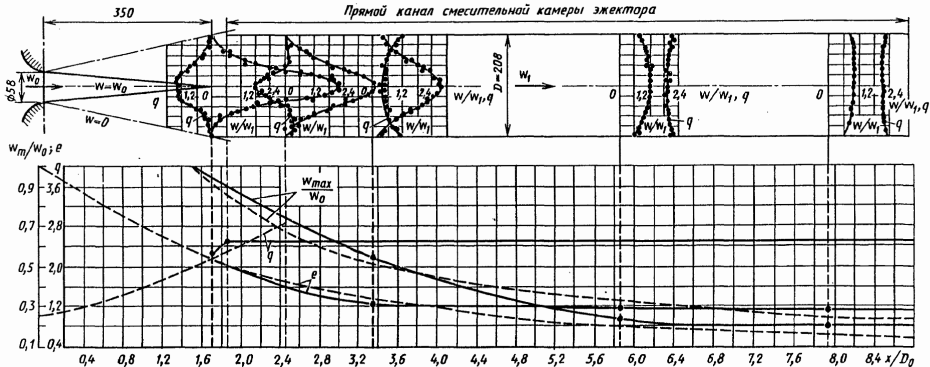
Рис. 4-6. Схемы распределения скоростей на основном участке свободной струи и после входа ее в смесительную камеру эжектора: штриховые линии — теоретические кривые для свободной струи; сплошные линии — экспериментальные кривые для струи в канале [4-15]; g \equiv \frac{(p-p_a)}{\rho w^2/2}
