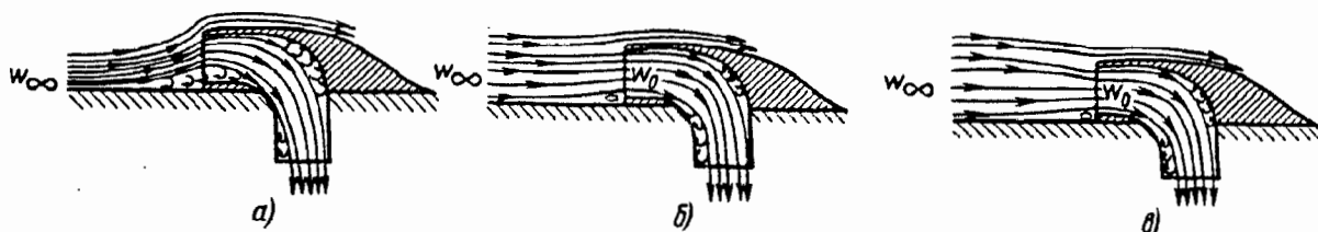
Рис. 3-9. Различные случаи входа потока в патрубок [3-11]:
