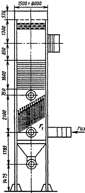
Центробежный скруббер ВТИ [12-25]
