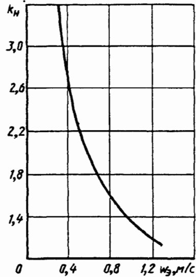
Рис. 12-5. Зависимость коэффициента k_{\text{к}} от w_0 при длине электрополя L=6 м и напряжении 45 кВ [12-87]
