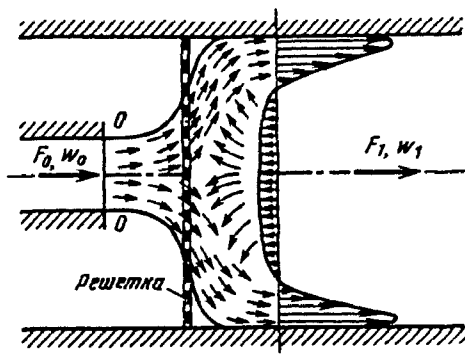
Рис. 8-7. Схема набегания узкой струи на решетку в трубе
