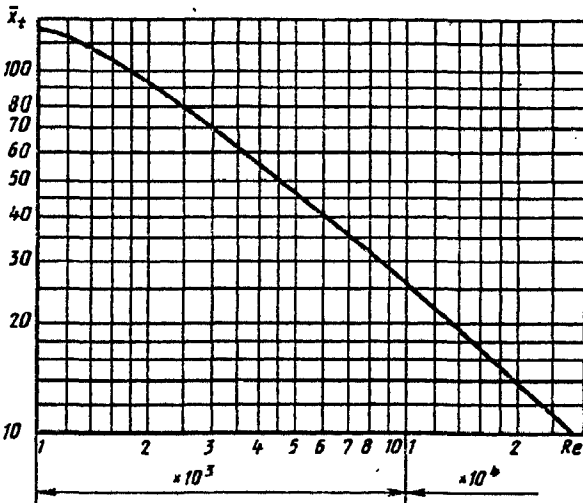
Рис. 1-6. Зависимость \bar{x}_t от Re
