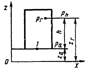
Рис. 1-8. Схема для определения давления в произвольной точке жидкости (газа) по давлению в заданной точке:
