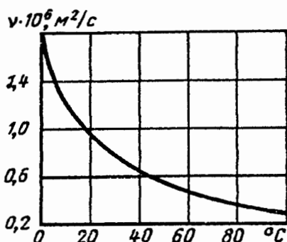
Рис. 1-2. Зависимость кинематической вязкости воды от ее температуры при 101,325 кПа
