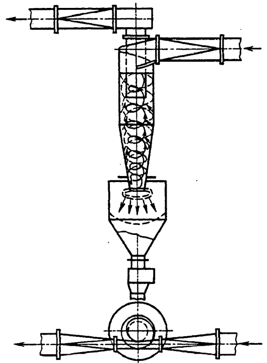
Рис. 12-2. Схема течения в корпусе циклона с раскручивающейся улиткой на выходе
