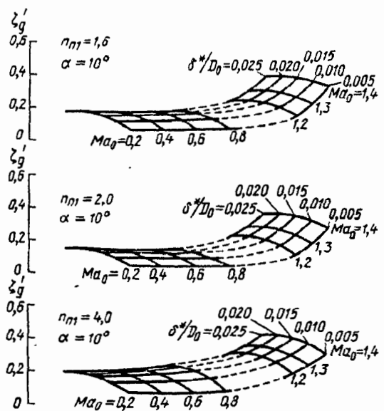
Рис. 5-18. Зависимость коэффициента сопротивления \zeta'_д диффузора с \alpha = 10^\circ от числа Маха ( Ma_0 ), условий входа ( \delta^*/D_0 ) и степени расширения ( n_{п1} ) [5-144]
