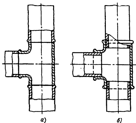
Рис. 7-7. Схема кольцевого выступа в стандартном тройнике:
