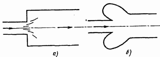
Рис. 4-7. Схемы участков с внезапным расширением сечения
