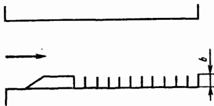
Рис. 4-8. Схемы участка с внезапным расширением сечения и с поперечными перегородками
