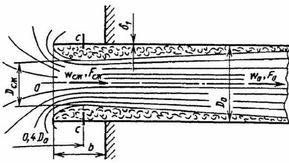
Рис. 3-1. Схема входа потока в прямую трубу из неограниченного пространства
