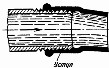
Рис. 6-13. Чугунные отводы, соединенные с помощью резьбы
