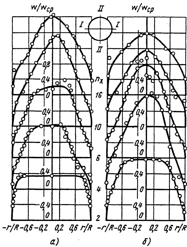
Рис. 5-3. Поля скоростей по диаметру I—I различных сечений (различных n_x ) конического диффузора при \alpha=8^\circ и Re=(4\div 5)\cdot 10^5 [5-54]: а— l_0/D_0=0 ; б— l_0/D_0=10
