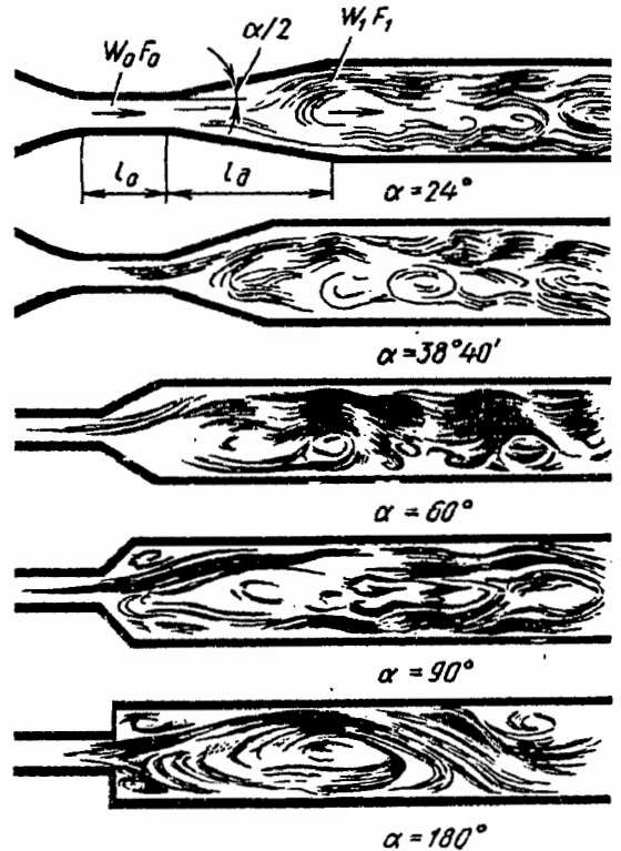
Рис. 5-1. Спектр потока в диффузорах с различными углами расширения при n_{\alpha 1} = F_1/F_0 = 3,3 [5-48]
