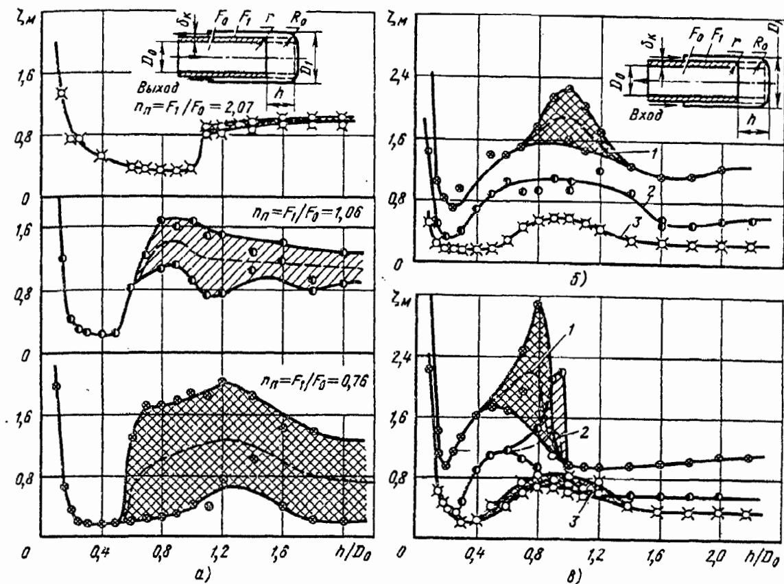
Рис. 6-21. Зависимость коэффициента сопротивления \zeta_m кольцевого поворота от h/D_0 при R/D_1=0,3 [6-19]: а — нагнетание при r/D_0=0,1 ; б — всасывание при r/D_0=0,2 ; 1 — n_\eta=0,80 ; 2 — n_\eta=1,07 ; 3 — n_\eta=2,1 ; в — всасывание при r/D_0=0,1 ; 1 — n_\eta=0,76 ; 2 — n_\eta=1,06 ; 3 — n_\eta=2,07
