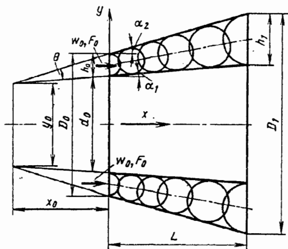
Рис. 5-26. Осекольцевой диффузор
