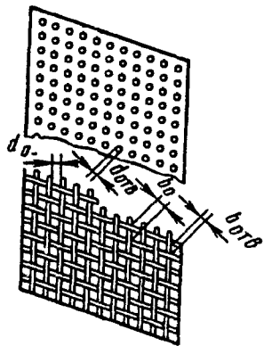
Решетки с различными формами краев отверстий, переходная и ламинарные области течения ( Re = \frac{w_0 d_r}{\nu} < 10^4 \div 10^5 ) [8-30]
