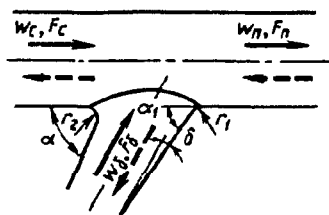
Рис. 7-5. Схема тройника улучшенной формы
