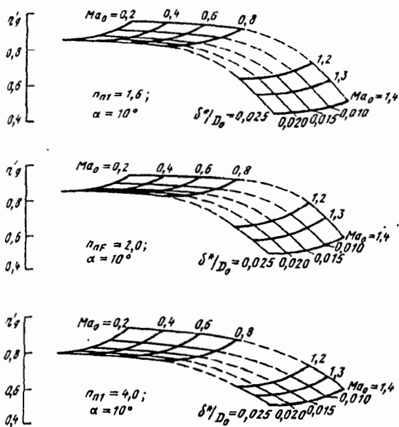
Рис. 5-17. Зависимость КПД диффузора \eta'_{1д} с \alpha = 10^\circ от числа Маха ( Ma_0 ), условий входа ( \delta^*/D_0 ) и степени расширения ( n_{п1} ) [5-144]
