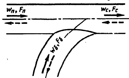
Рис. 7-6. Схема тройника с плавным отводом
