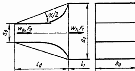
Диффузор плоский
