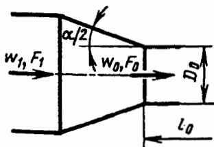
Конфузоры круглого сечения в сети ( l_0/D_0 > 0 ); ламинарный режим течения Re = w_0 D_r / \nu \leq 50 [5-4]
