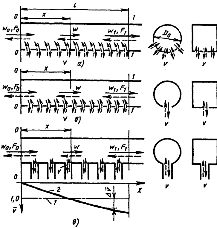
Рис. 2-7. Схемы течения жидкости в коллекторах с изменением расхода вдоль пути; коллекторы: а — с перфорированными стенками; б — с продольной щелью; в — с боковыми ответвлениями: 1 — \bar{v} = 1,0 = \text{const} ; 2 — \bar{v} при переменном оттоке
