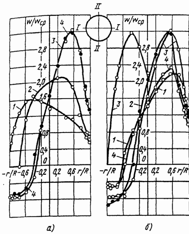
Рис. 5-7. Поля скоростей в коническом диффузоре при \alpha=20^\circ по сечению n_x=4 при Re=(4\div 5)\cdot 10^5 и различных l_0/D_0 [5-54]: а—диаметр I—I; б—диаметр II—II; 1— l_0/D_0=0 ; 2— l_0/D_0=5 ; 3— l_0/D_0=10 ; 4— l_0/D_0=20
