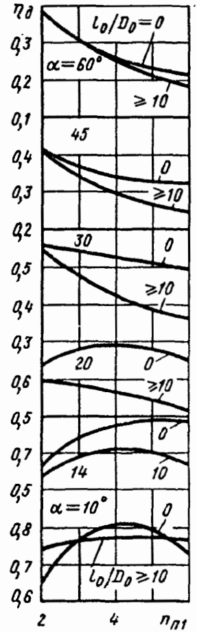
Рис. 5-16. Зависимость \eta_d от n_{\pi 1} для плоского диффузора
