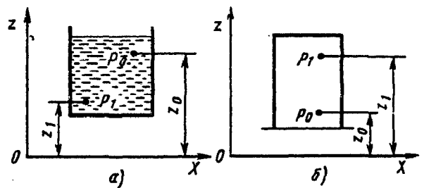
Рис. 1-8. Схема для определения давления в произвольной точке жидкости (газа) по давлению в заданной точке:
