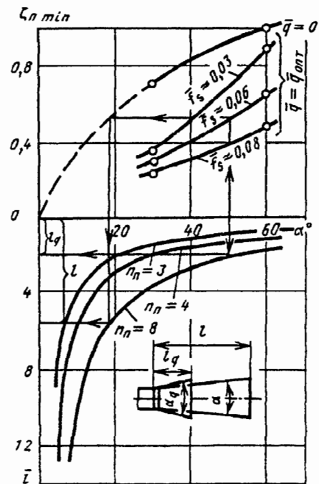
Рис. 5-22. Сводная зависимость минимальных потерь полного давления от площади щели при различных углах раскрытия диффузора и сдувании пограничного слоя [5-95]
