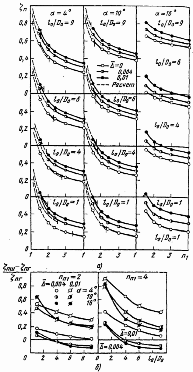
Рис. 5-12. Зависимость сопротивления диффузоров от шероховатости \bar{\Delta} [5-14]: а — \zeta_n = f(n_{п1}, \alpha, l_0/D_0, \bar{\Delta}) ; б — (\zeta_{n,ш} - \zeta_{n,r}) / \zeta_{n,r} = f(l_0/D_0, n_{п1}, \bar{\Delta})
