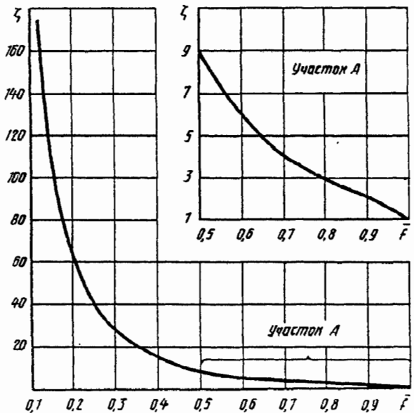
Выход из прямой трубы через шайбу или плоскую решетку; с острыми краями отверстий ( l/d_r = 0 \div 0,015 ); Re = w_{отв} d_r / \nu \geq 10^5 [11-16—11-18]
