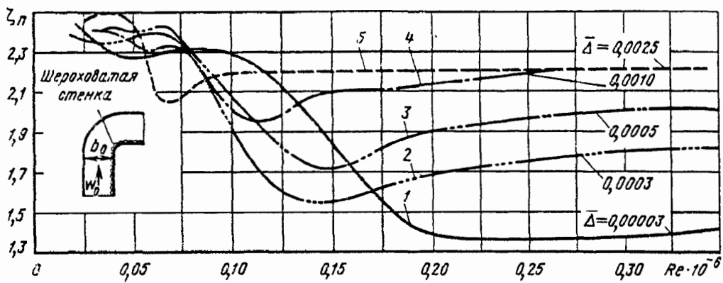
Рис. 6-9. Кривые сопротивления \zeta_{\text{п}} = f(\text{Re}) отвода, с внутренней стенкой [6-17]: 1—гладкой; покрытой: 2—оберточной бумагой; 3—афишной тишеной бумагой; 4—шлифовальной шкуркой № 140; 5—шлифовальной шкуркой № 60
