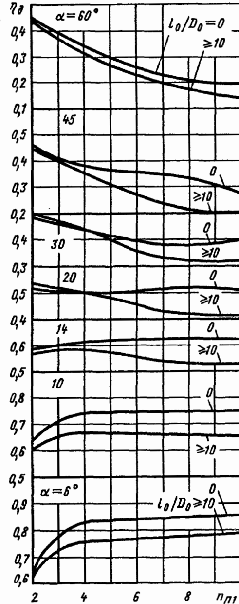
Рис. 5-14. Зависимость \eta_d от n_{\pi 1} для конического диффузора
