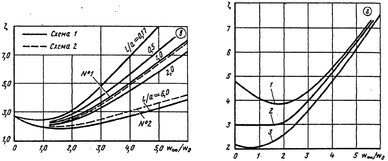
Значения \zeta для схемы 3 (график z)
