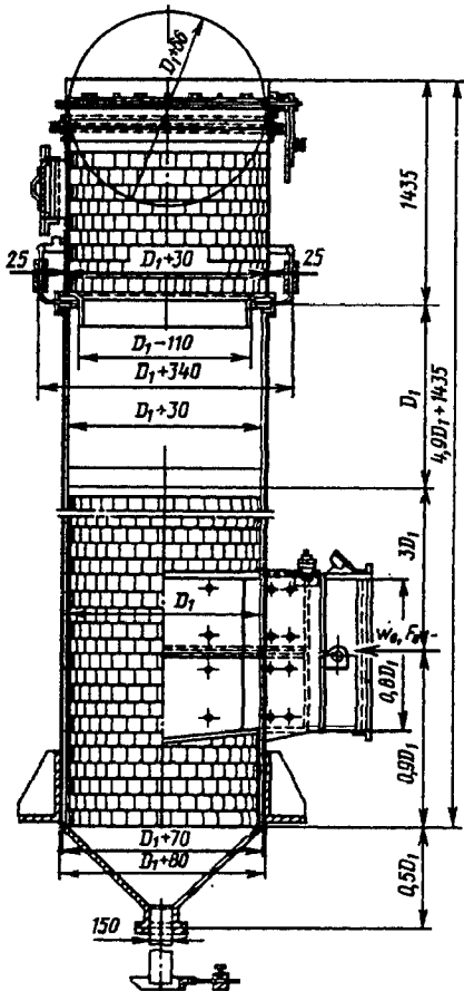
Центробежный скруббер ВТИ [12-25]
