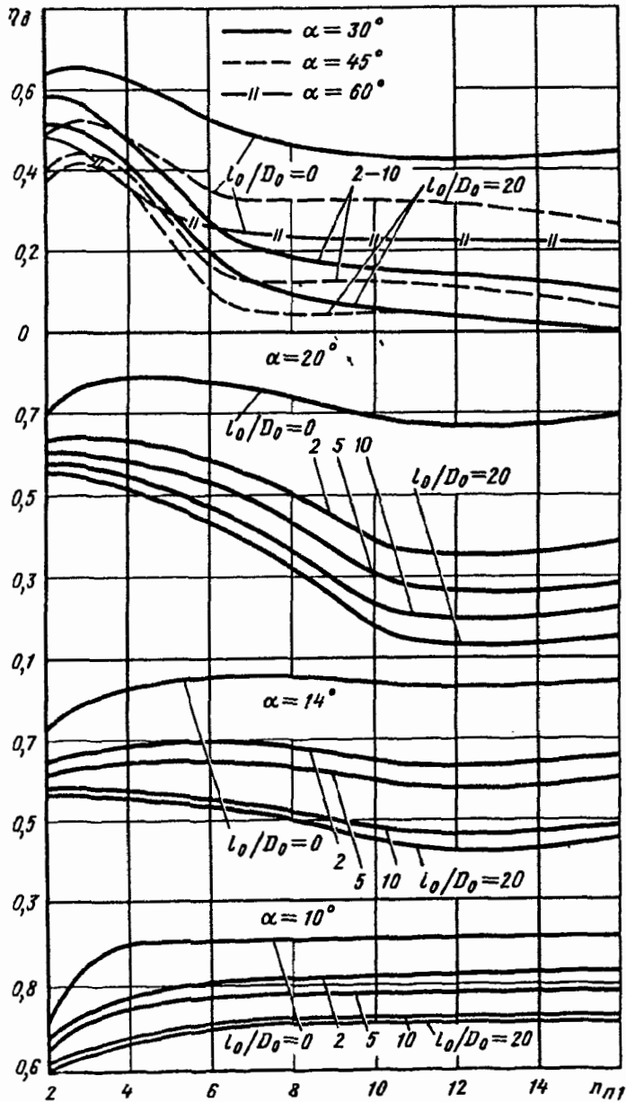
Рис. 5-14. Зависимость \eta_d от n_{\pi 1} для конического диффузора
