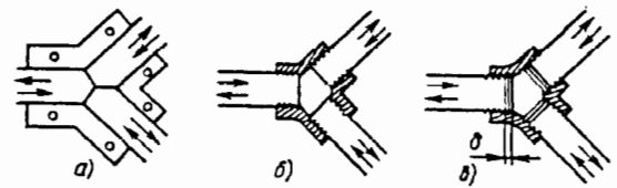
Рис. 7-9. Тройники симметричной формы типа F_6 = F_n = F_c [7-57]:
