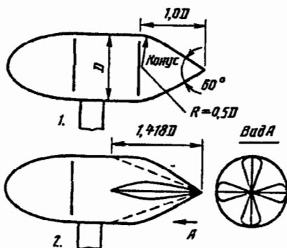
Рис. 10-7. Схема плохообтекаемых тел вращения [10-32]:
