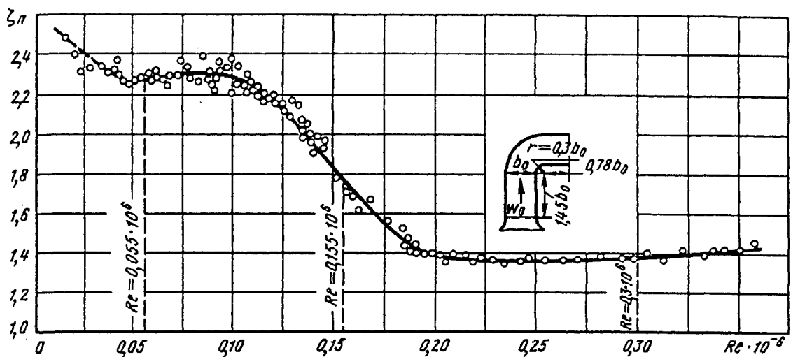
Рис. 6-7. Зависимость коэффициента полного сопротивления \zeta_{л} от числа Re для отвода с \delta=90^\circ и гладкими стенками ( \Delta=0,00003 ) [6-17]
