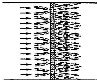
Рис. 8-1. Схема перетекания потока через решетку (сетку)
