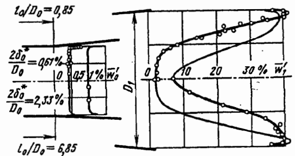
Рис. 5-10. Изменение продольной пульсационной скорости \bar{w}' = w'/w_0 во входном сечении диффузора с изменением относительной длины прямого входного участка l_0/D_0 [5-172, 5-173]
