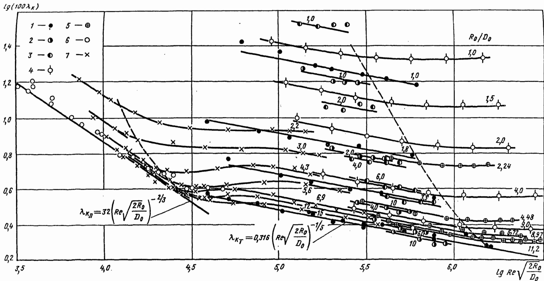
Рис. 6-5. Коэффициент сопротивления \lambda_{\kappa} плавных поворотов на 90^\circ в функции безразмерного параметра Re\sqrt{2R_0/D_0} [6-56]: 1—Ито, D_0=35 мм, латунь; 2—Гофман, D_0=43 мм, латунь; 3—Гофман, D_0=43 мм, латунь шероховатая; 4—Цимерман, D_0=50 мм, сталь; 5—Грегорики, D_0=89,3 мм, сталь; 6—Идельчик, гладкие; 7—Ли, D_0=20 мм, сталь
