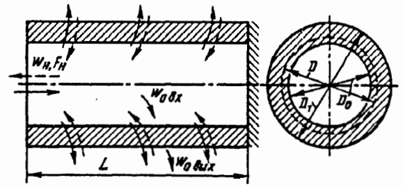
Рис. 8-5. Слоевой (пористый) цилиндр
