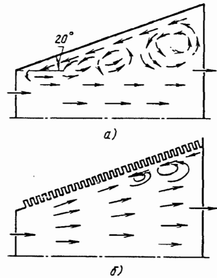
Рис. 5-25. Схема течения потока в диффузоре [5-61, 5-62]:
