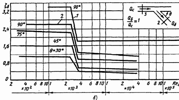
Рис. 7-8. Зависимость коэффициентов сопротивления \zeta_\delta тройников от числа Re [7-8]: а — вытяжные тройники; б — приточные тройники
