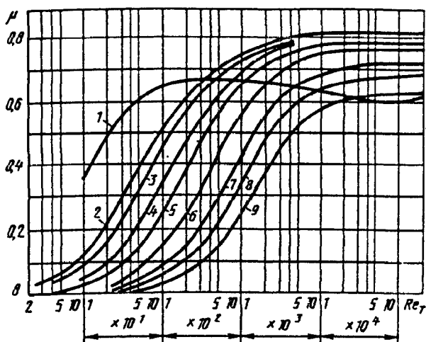
Рис. 1-18. Зависимость коэффициента расхода при истечении из наружных цилиндрических насадок от числа Рейнольдса Re_{\tau} [1-55]:
