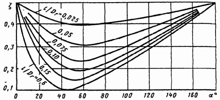
Значения \zeta (приближенно)
