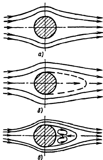
Рис. 10-2. Спектры потока в следе за сферическим телом при различных режимах обтекания в пределах малых и умеренных чисел Рейнольдса: а — Re' \leq 1 ; б — 0,05 < Re' < (5 \div 10) ; в — (5 \div 10) < Re' < (40 \div 50)
