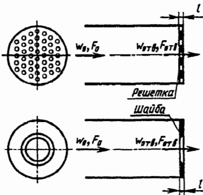
Выход из прямой трубы через шайбу или плоскую решетку; с острыми краями отверстий ( l/d_r = 0 \div 0,015 ); Re = w_{отв} d_r / \nu \geq 10^5 [11-16—11-18]
