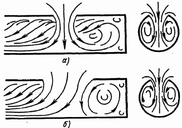
Рис. 3-6. Схемы входа потока в боковое отверстие концевой участка трубы: а—при малых значениях \bar{f} ; б—при больших значениях \bar{f}
