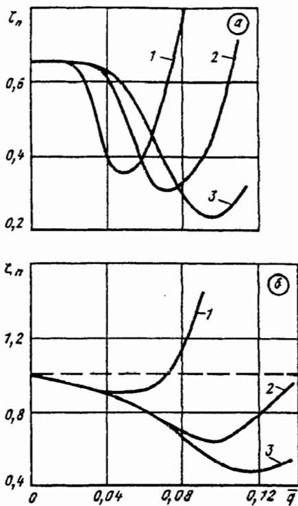
Рис. 5-21. Зависимость \zeta_n от \bar{q} при сдувании пограничного слоя [5-95]:
