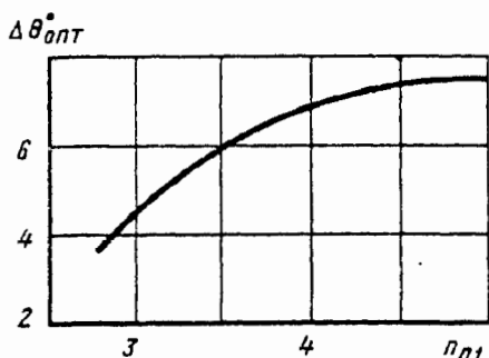
Рис. 5-23. Зависимость угла \Delta\theta_{\text{опт}} от степени расширения n_{п1} [5-96]
