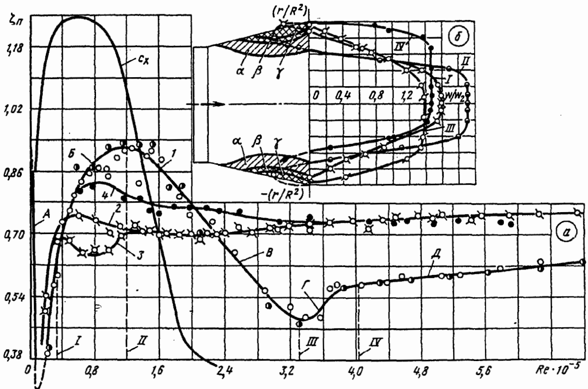
Рис. 5-11. Зависимость \zeta_n = f_1(Re) и c_x = f_2(Re) (а) и поля скоростей по сечению n_x=2 в коническом диффузоре при \alpha=30^\circ , n_{n1}=2 и l_1/D_1=0 (б) [5-54]: I— Re=0,3 \cdot 10^5 ; II( \alpha )— Re=1,2 \cdot 10^5 ; III( \beta )— Re=3,3 \cdot 10^5 ; IV( \gamma )— Re=4 \cdot 10^5 ; 1— l_0/D_0=0 ; 2— l_0/D_0=2 ; 3— l_0/D_0=3 с турбулизатором; 4— l_0/D_0=20
