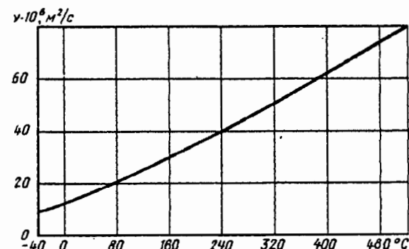
Рис. 1-1. Зависимость кинематической вязкости воздуха от его температуры при давлении 101,325 кПа
